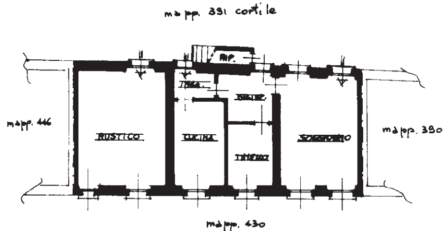
PIANTA PIANO TERRA H=270
