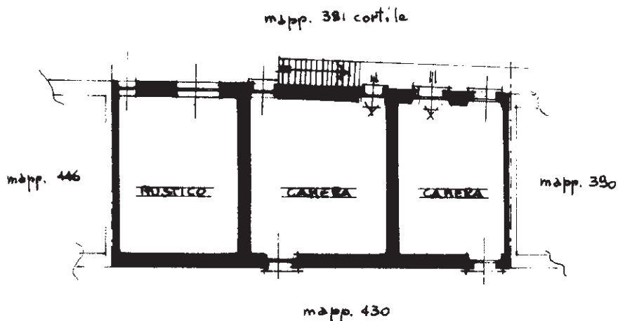
PIANTA PIANO PRIMO H=270
